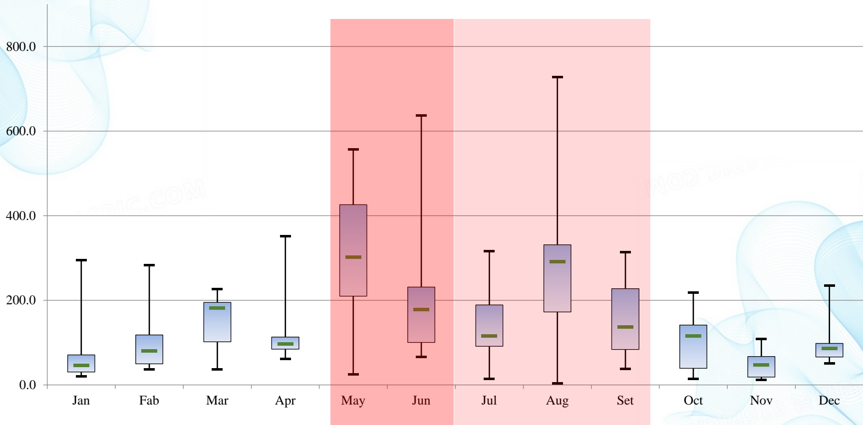
桃園市2013~2023降雨量/月平均圖
